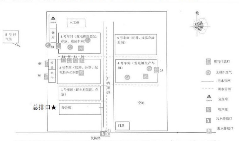
附图 3-2-1 本项目调整后厂区平面布置图
