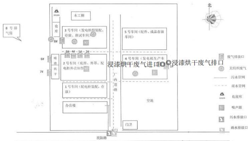
附图 3-2-1 本项目调整后厂区平面布置图
